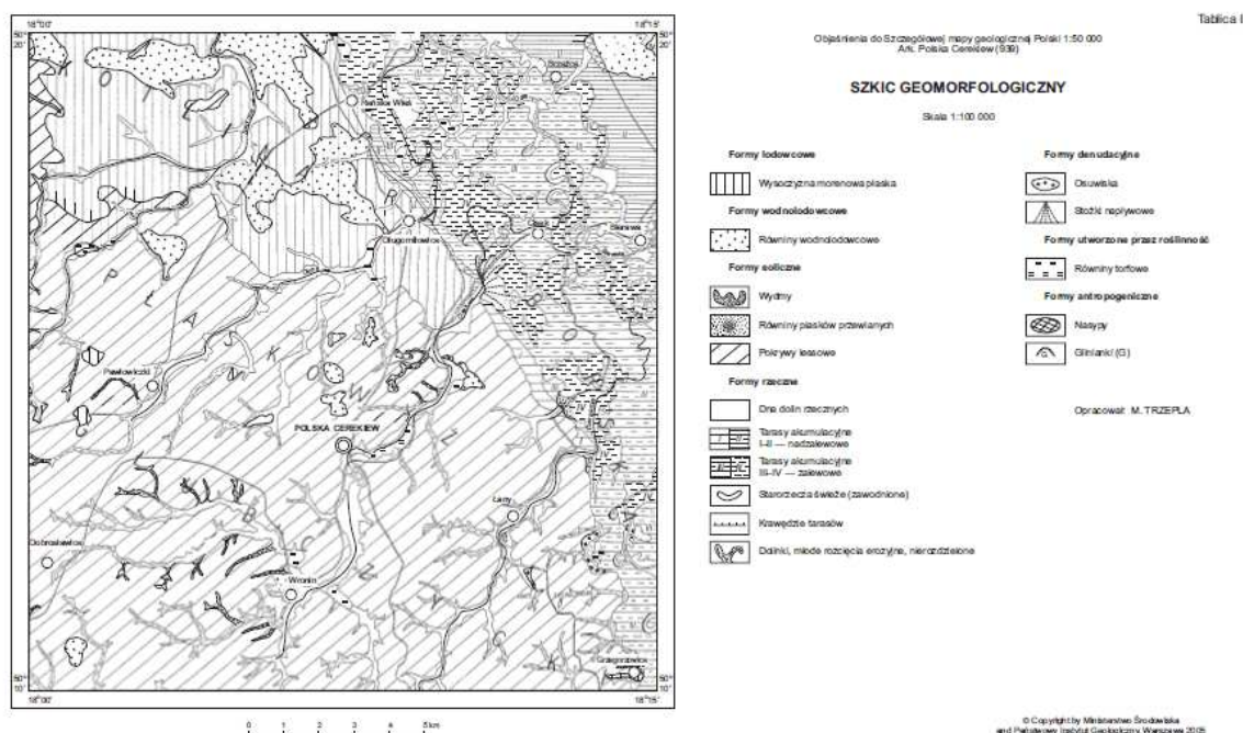
Ryc. 1. Szkic geomorfologiczny obejmujący rejon zmiany studium (źródło: Objasnienia do szczegółowej mapy geologicznej Polski, ark. Polska Cerekiew, PIG, Warszawa, 2005).
