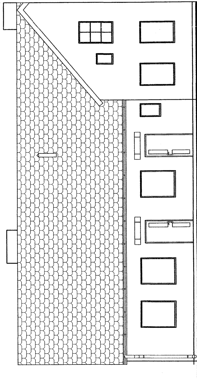
ELEWACJA POŁUDNIOWO - WSCHODNIA
