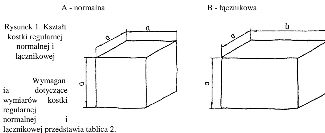
Tablica 2. Wymiary kostki regularnej normalnej i łącznikowej oraz dopuszczalne odchyłki
